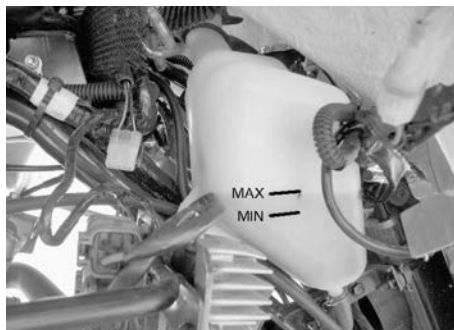
NIVEAU DE LIQUIDE DE REFOUDDISSEMENT
