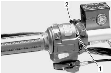
TIPIQUE – INTERRUPTEUR D'ARRÊT D'URGENCE DU MOTEUR
