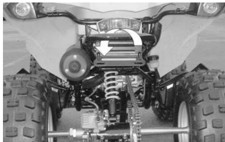
POINT D'ARRIMAGE DES SANGLES AU PARE-CHOC ARRIÈRE
