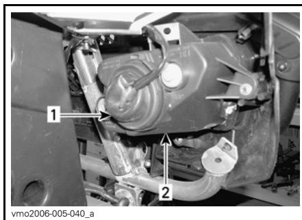
1. Gummischutz 2. Scheinwerfergehäuse
