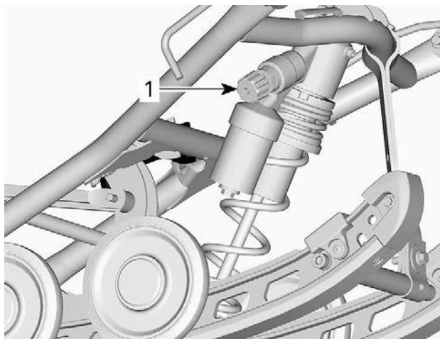
1. Justerknopp för centralstötdämparens kompressionstrykdämpning
