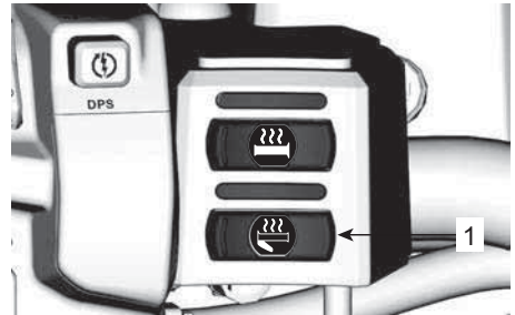
1. Schalter für beheizbaren Gashebel
