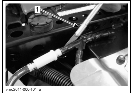
TYPBILD - KAPA SLANG FÖRSIKTIGT
