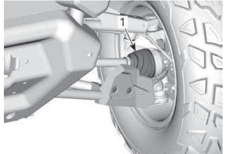
1. Balg buitenkant aandrijftras
