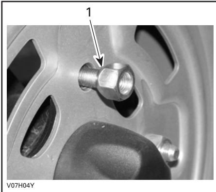
TÍPICA - RODA DE AÇO 1. Lado cônico da porca (tipo passante)
