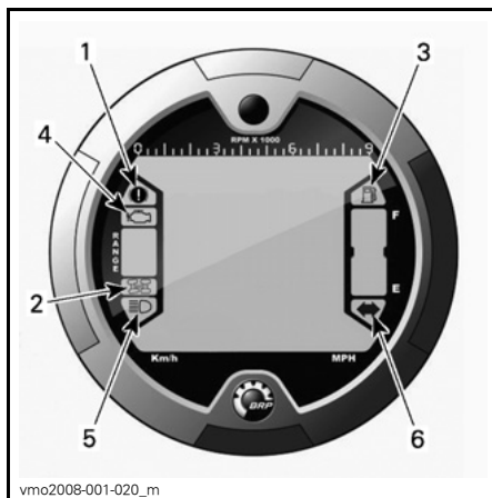
1. Luz indicadora do freio 2. Lâmpada indicadora do 4WD 3. Luz indicadora de nível de combustível baixo 4. Luz indicadora de problema no motor 5. Luz indicadora de farol alto 6. Luz indicadora de seta/pisca-alerta
