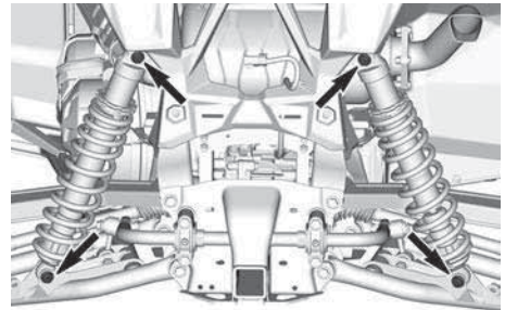
ТИПОВОЙ ВАРИАНТ — КРЕПЕЖНЫЕ ДЕТАЛИ ЗАДНЕГО АМОРТИЗАТОРА
