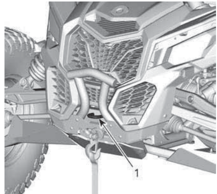
1. Vorderer Abschlepphaken
