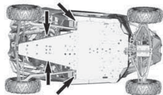
WAGENHEBERSTÜTZBOCK FAHRZEUGHECK
