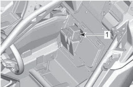
1. Hinterer Sicherungskasten
