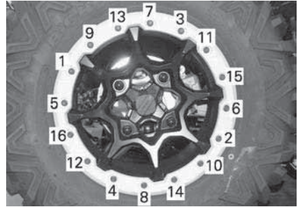
TYPISCH – ANZIEHREIHENFOLGE
