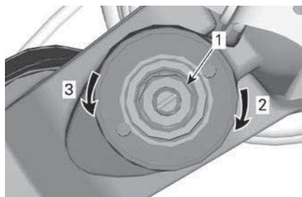
COMPRESSIEDEMPING BIJ HOGE SNELHEID (GEBRUIK EEN SLEUTEL VAN 17 MM)
