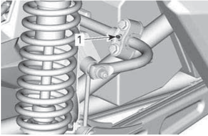
TYPISCH ACHTERAAN - STABILISATIESTANG
