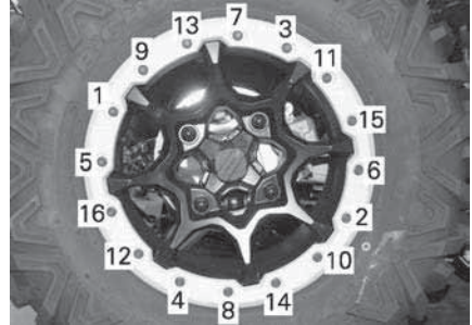
TYPISCH - AANDRAAIVOLGORDE
