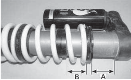
TYPISCH - BIJSTELLING CROSSOVER - ACHTERSCHOKDEMPEM
