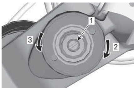
COMPRESSIEDEMPING BIJ LAGE SNELHEID (GEBRUIK EEN SCHROEVENDRAAIER)
