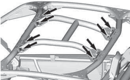
CENTRALE VERSTERKING
