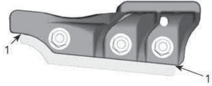
1. Verschleißgrenze
