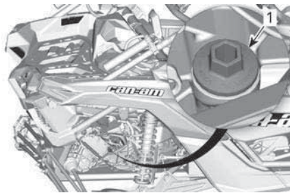
1. Getriebeöl-Füllstand-Verschlusskappe
