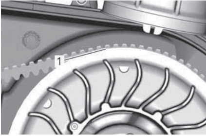
1. Unterster Teil der Zahnräder bündig mit der Abtriebsscheibenkante
