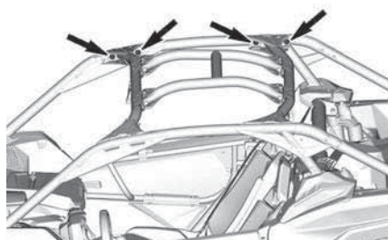
ПРАВЫЙ БОКОВОЙ КАРКАС БЕЗОПАСНОСТИ
