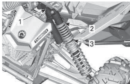
ТИПОВОЙ ВАРИАНТ - БЕЗ ДЕМПФИРОВАНИЯ ХОДА ОТБОЯ - ПЕРЕДНЯЯ ПОДВЕСКА
