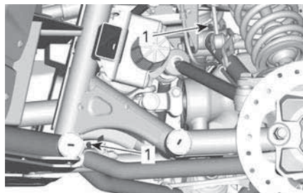
TYPISCH - VOOROPHANGING
