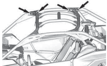
JAULA LATERAL DEL LADO DERECHO
