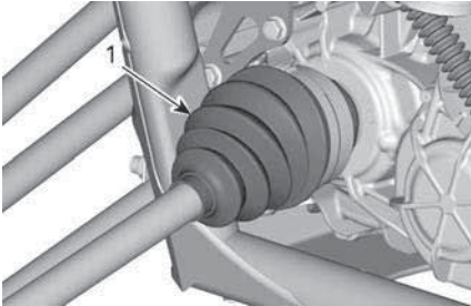
PARTE TRASERA DEL VEHÍCULO (COMPONENTES DESMONTADOS PARA MAYOR CLARIDAD)
