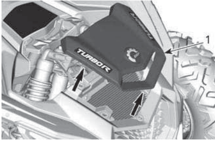
TAPA DE PROTECCIÓN
