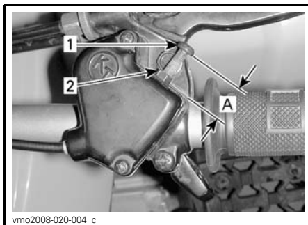
1. Vis de limiteur de régime 2. Écrou de blocage A. Réglage maximal de la course de la manette d'accélérateur 20 mm
