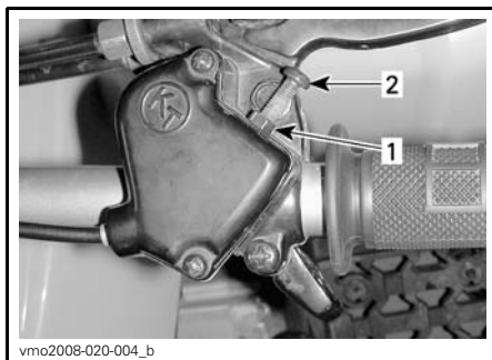
1. Écrou de blocage 2. Vis de limiteur de régime
