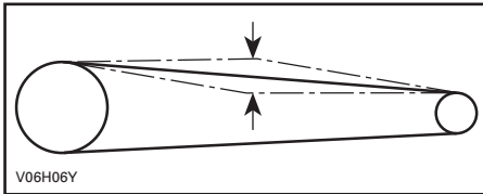
FLÈCHE DE LA CHAÎNE D'ENTRAÎNEMENT ENTRE 15 MM ET 25 MM
