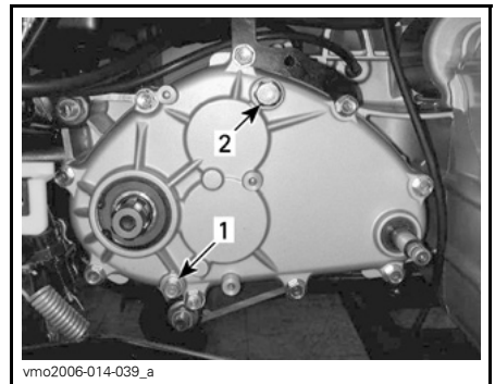
1. Aftapplug tandwielkast
