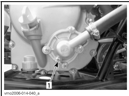
1. Aftapplug van het koelsysteem
