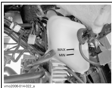
KOELVLOEISTOFPEIL
