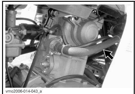
PLAATS SLANGKLEM
