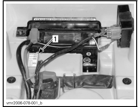
1. Portafusibles
