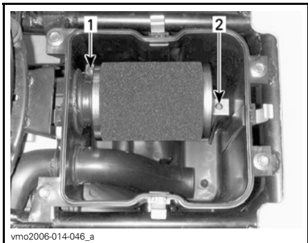
TÍPICO - ROCÍE EL ELEMENTO DE FILTRO POR DENTRO Y POR FUERA.
