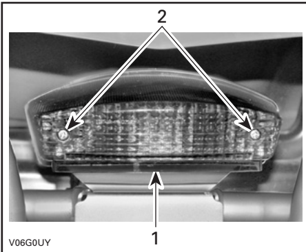
1. Lente 2. Tornillos
