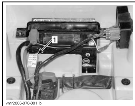
1. Porte-fusibles
