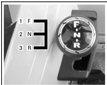
PAUTA DE LA PALANCA DE TRANSMISIÓN
