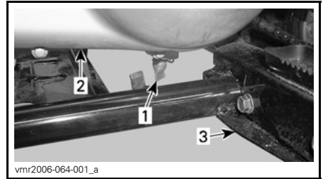
1. Tubo de vaciado de la cubierta de la CVT 2. Tapa de CVT 3. Estribo izquierdo
