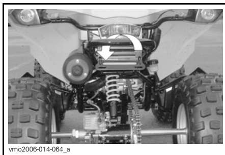
TÍPICO – UBICACIÓN DE LA CORREA EN EL PARACHOQUES TRASERO
