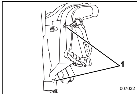
1. Punti di lubrificazione leva di ribaltamento e staffa del supporto girevole (annuale)
