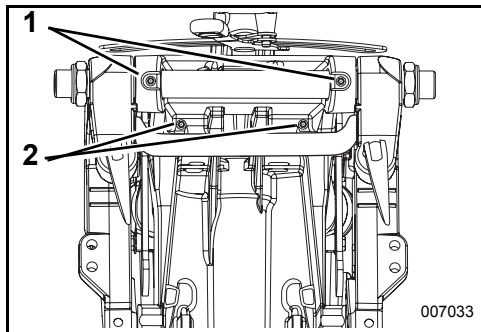
1. Punti di lubrificazione del tubo di ribaltamento (annuale) 2. Asse leva ribaltamento (annuale)
