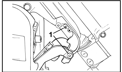
1. Σημεία λίπανσης μοντέλων με υδραυλικό σύστημα διαγωγής και ανύψωσης, στηρίγματος τοποθέτησης σε τρέιλερ και περιστροφικού στηρίγματος (κάθε χρόνο)
