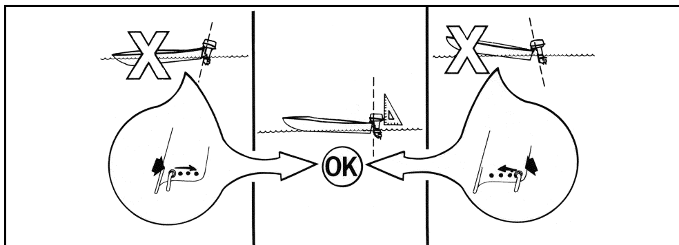
Ρύθμιση της γωνίας της εξωλέμβιας
