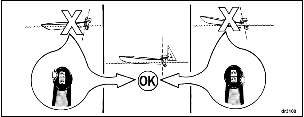
Ρύθμιση γωνίας διαγωγής
