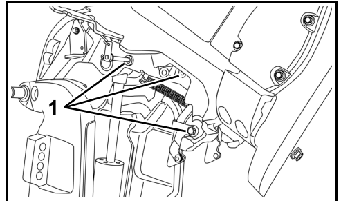
1. Σημεία λίπανσης μοντέλων με μη αυτόματο σύστημα ανύψωσης, περιστρεφόμενου στηρίγματος (κάθε χρόνο)
