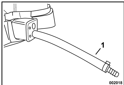
1. Εύκαμπτος σωλήνας και σύνδεσμος παροχής καυσίμου – 9 mm (3/8")
