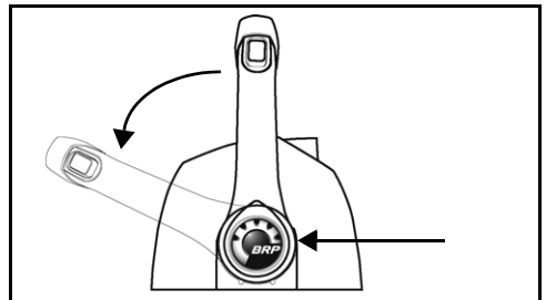
Χειριστήριο τύπου Binnacle - Συνήθης
