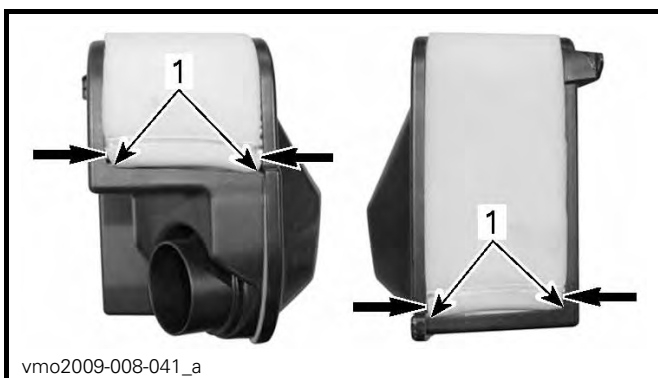
1. Skumfilterelementets ytterkanter
