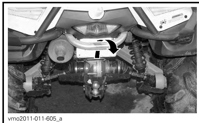
TYPBILD- FÄSTPUNKT FÖR BAKRE FÄSTREMMAR
