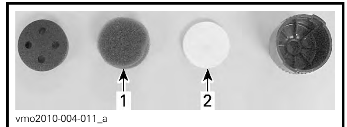
ACS-KOMPRESSORNS LUFTFILTER AVLÄGSNAT FÖR TYDLIGHETENS SKULL
