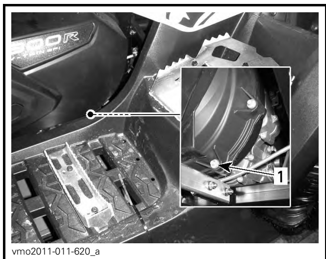
NÄRA VÄNSTER FOTSTÖD 1. Tömningsskruv
