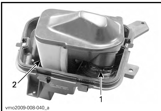
TYPBILD 1. Klämman 2. Luftfilter
