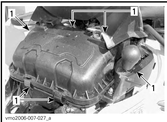
1. Frigör klämmorna
