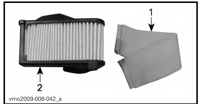
1. Skumfilterelement 2. Pappersfilter
