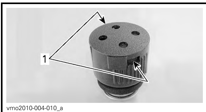
ACS-KOMPRESSORNS LUFTFILTER AVLÄGSNAT FÖR TYDLIGHETENS SKULL 1. spärrhakar
