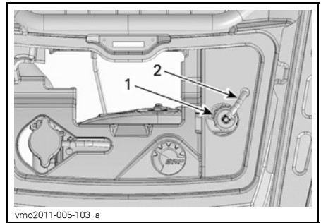
TYPISCH 1. Einfüllkappe 2. Schlauch des Kühlmittelbehälters
