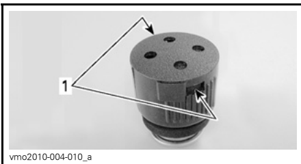
ACS-KOMPRESSOR-LUFTFILTER ZUR VERDEUTLICHUNG ENTFERNT 1. Rastungen
