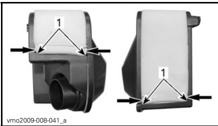
1. Äußere Enden des Schaumstofffilterelements
