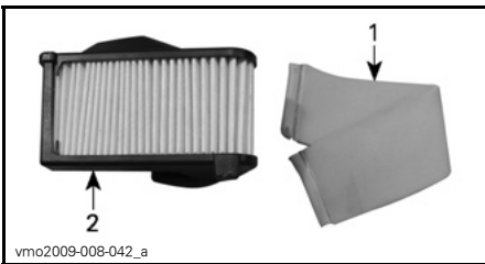
1. Schaumfilterelement 2. Papierfilter
