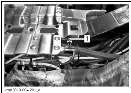
1. Anschlussstück des Kompressors
