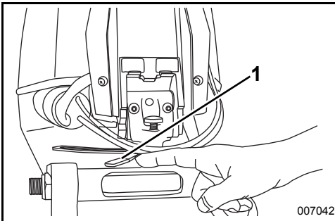
1. Styrefriksjonsspak
