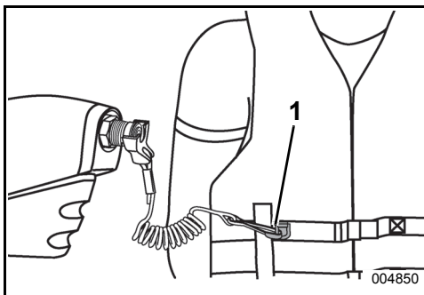
1. Utløpersnor
