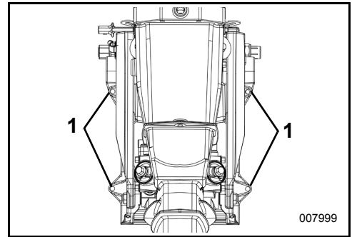
1. Borede hull i akterspeil, 15 HO-modeller
