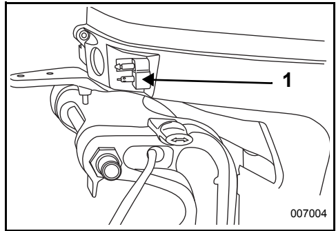
1. Drivstoffkopligen
