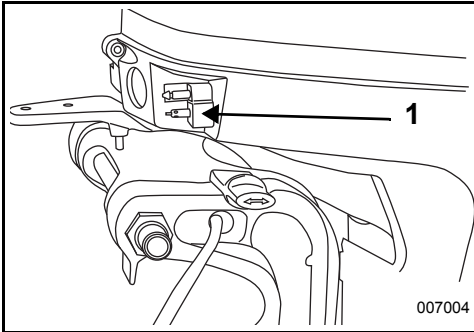
1. Drivstoffkoping
