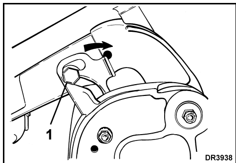
1. Levier de support de relevage – en position DÉVERROUILLÉE
