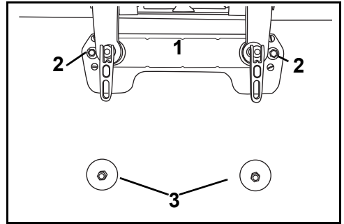
1. Plaque de tableau arrière 2. Petites rondelles 3. Grandes rondelles
