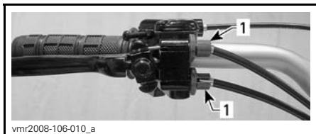
1. Justeringsskruvar på handtaget
