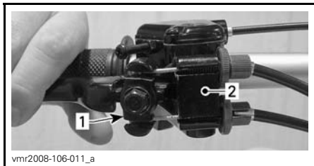
1. Vajerlänk 2. Vajerfäste
