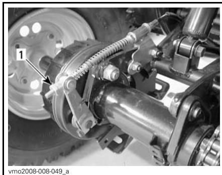
1. Bromsvajerns justerskrub
