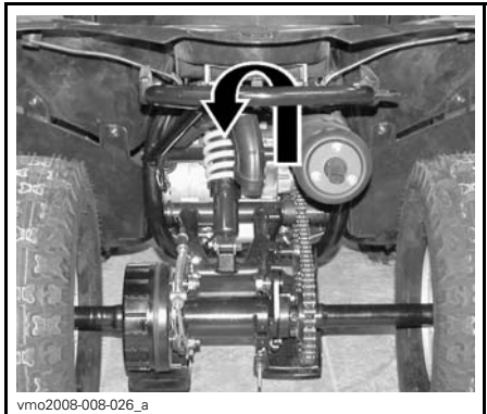
ALLA MODELLER — FÄSTPUNKT FÖR BAKRE FÄSTREMMAR
