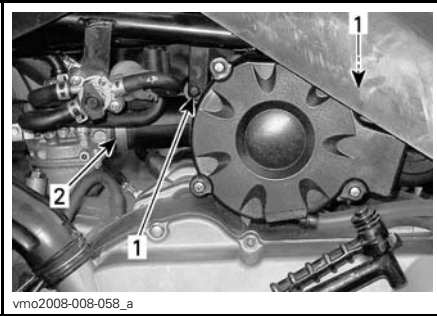
1. Ilmansuodattimen kotelo
