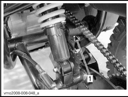
1. Voimansiirtoketjun rulla
