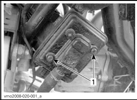
1. Irrota ruuvit
