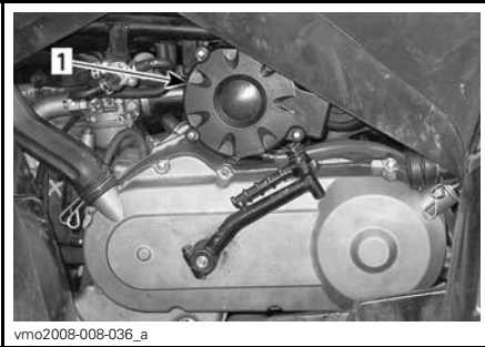
1. Ilmansuodattimen kotelo
