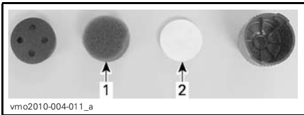
FILTRE À AIR DU COMPRESSEUR ACS RETIRÉ POUR PLUS DE CLARTE
