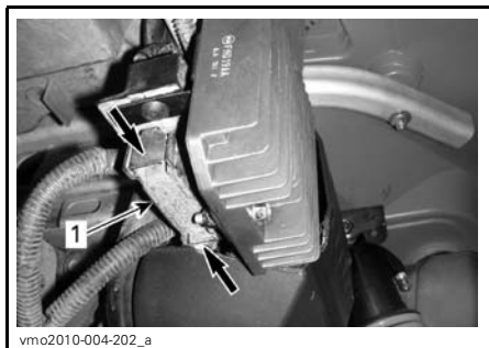
TYPIQUE - VUE DU OUTLANDER 800R LTD 1. Porte-fusibles arrière
