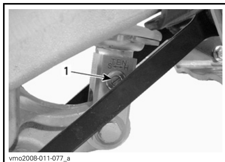
1. Regelaar terugvering (platte schroevendraaier)
