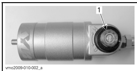
1. Compressieregelaar hoge snelheid (sleutel van 17 mm)
