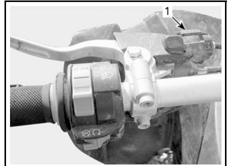
1. Kabelstelschroef
