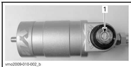
1. Regelaar compressie bij lage snelheid (platte schroevendraaier)
