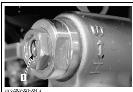
vmo2008-021-004_a 1. Regelaar compressie bij lage snelheid (platte schroevendraaier)
