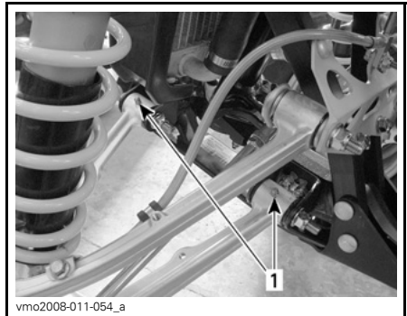
vm02008-011-054_a TYPISCH — ONDERSTE WIELDRAAGARM 1. Smeerfittingen
