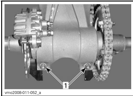
1. Borgbouten achteras
