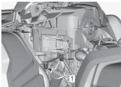
1. Luftfilter-Ablassrohr Motorluftfilter reinigen und ölen
