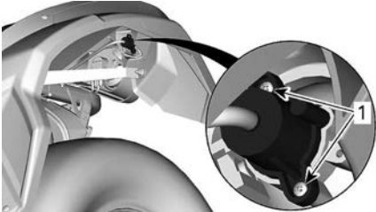
代表例 - リア方向指示灯
