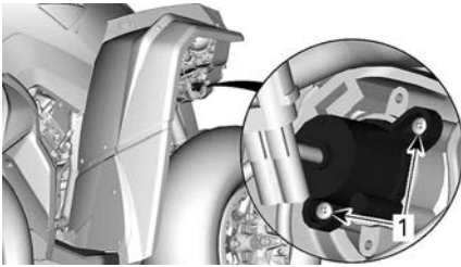
代表例 - フロント方向指示灯
