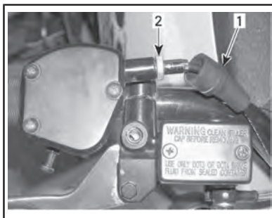
1. Protetor de borracha 2. Ajuste do cabo
