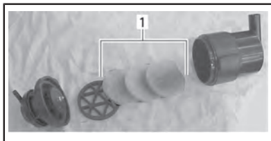
1. Filtros
