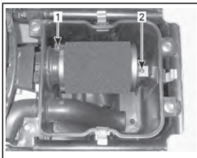
1. Braçadeira
