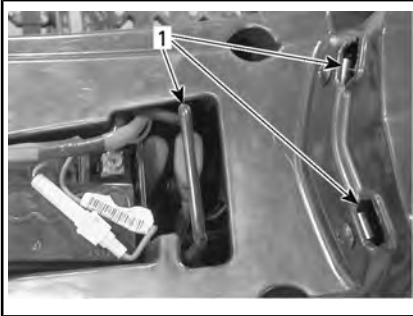
1. Петли
