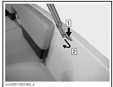
Fase 1: Premere il dispositivo di blocco Fase 2: Far scorrere il telaio del Bimini top verso l'esterno
