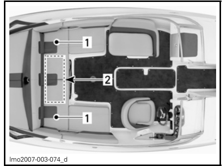
Imo2007-003-074_d CHALLENGER 230 1. Vano bagagli 2. Coperchio di accesso del vano motore
