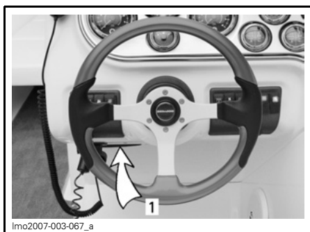
1. Posizione fusibili
