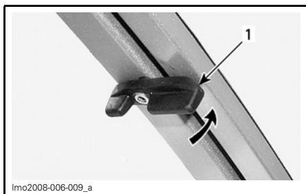
SITUAZIONE TIPICA — ENTRAMBI I LATI 1. Blocco parabrezza
