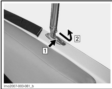
Fase 1: Premere il dispositivo di blocco Fase 2: Far scorrere il montante di supporto verso l'esterno
