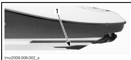
SITUAZIONE TIPICA — ENTRAMBI I LATI 1. Ingressi dell'acqua pompa a getto
