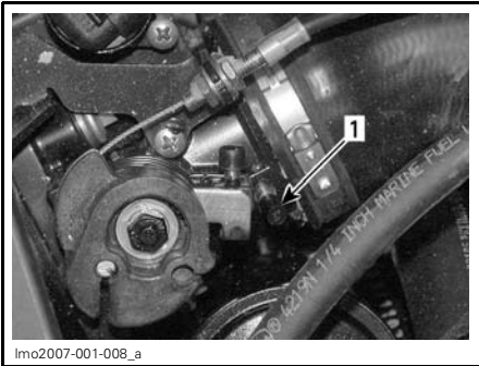
ENLEVER LE CAPUCHON 1. Capuchon de plastique
