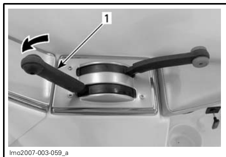
1. Levier sélecteur en position «marche avant»
