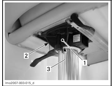
TYPIQUE 1. Film de graisse 2. Moyeu de la pièce coulée 3. Coupelle
