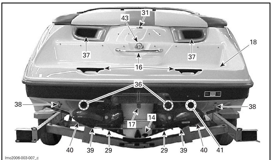
TÍPICO — VISTA TRASEIRA
