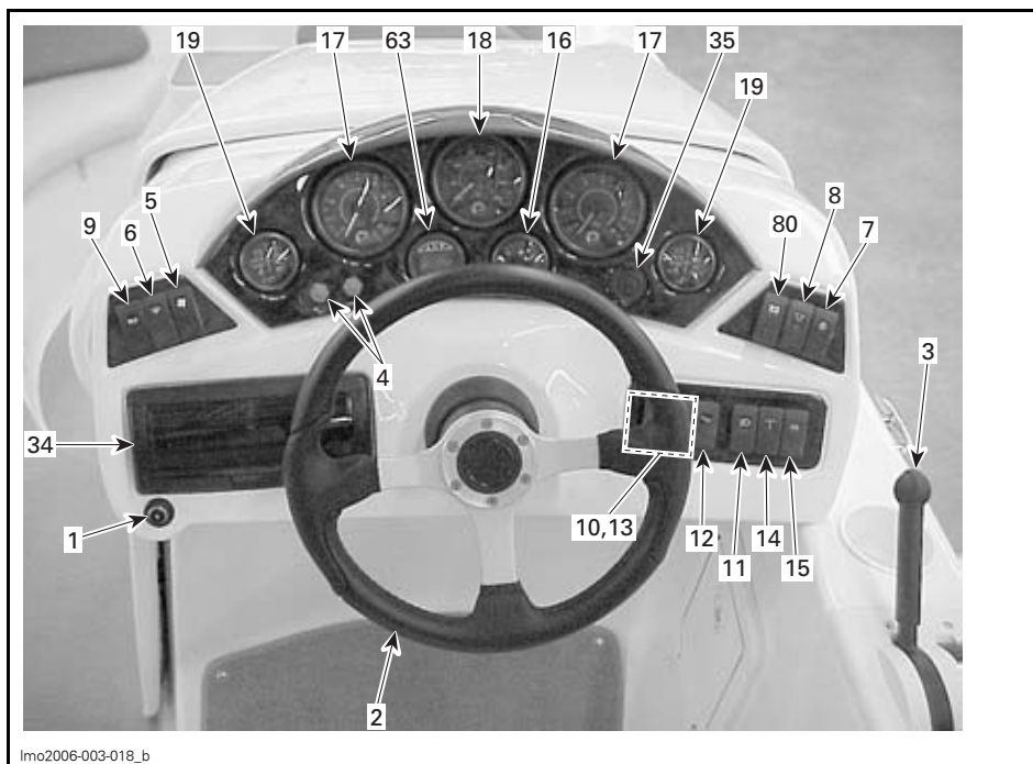
VISTA DE LA CABINA DE MANDO — 220 ISLANDIA SE
