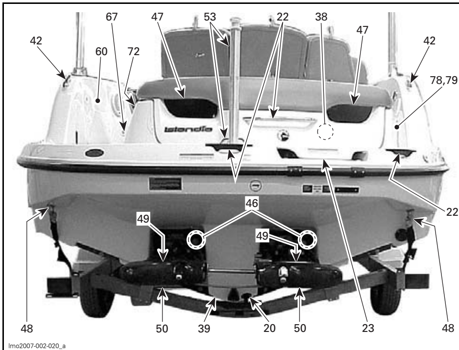
TÍPICO — VISTA POR POPA — 220 ISLANDIA SE
