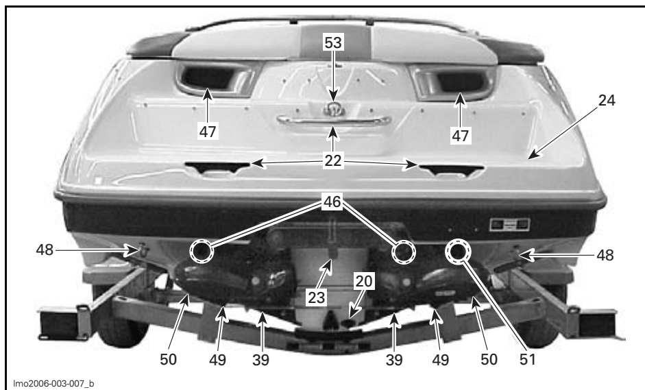
TÍPICO — VISTA POR POPA — 205 UTOPIA
