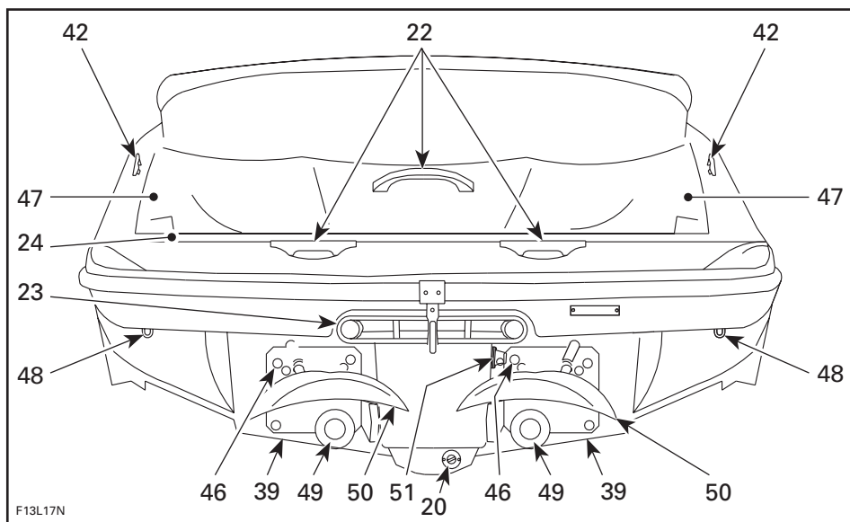
TÍPICO — VISTA POR POPA — 200 SPEEDSTER
