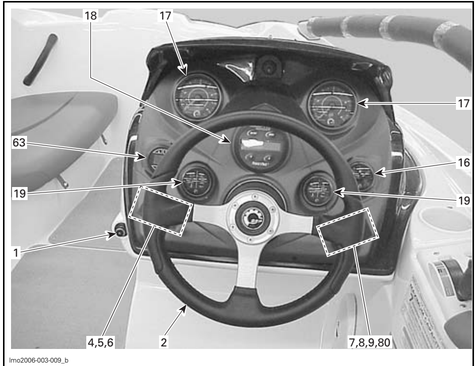
VISTA DE LA CABINA DE MANDO — 200 SPEEDSTER
