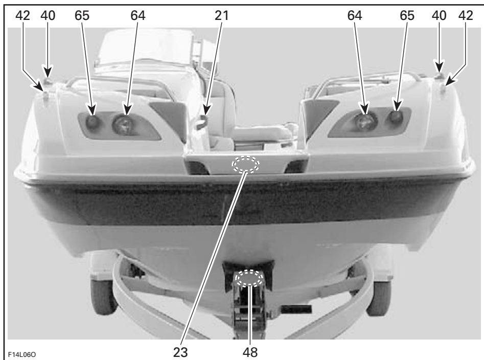
TÍPICO — VISTA POR PROA — 220 ISLANDIA SE
