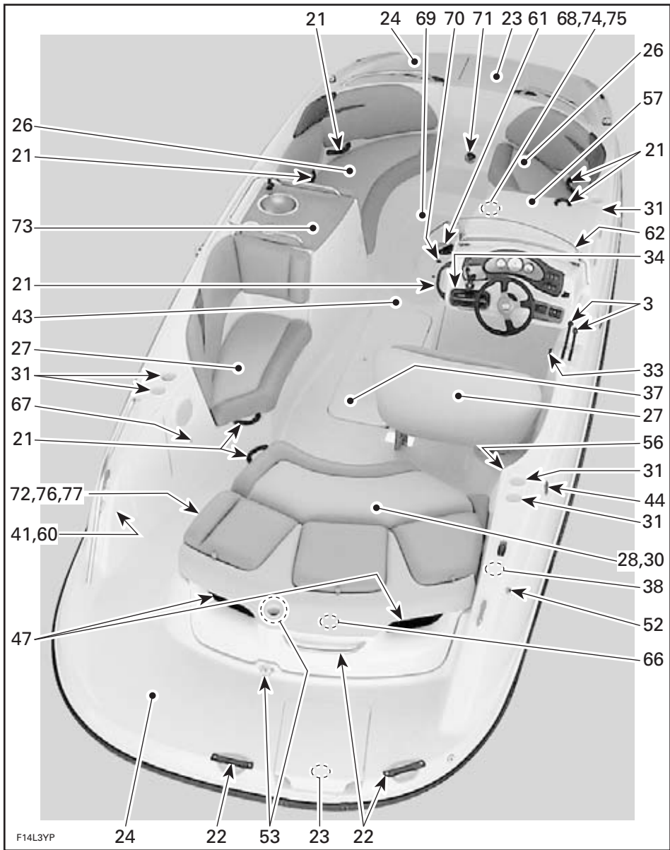
TÍPICO — 220 ISLANDIA SE
