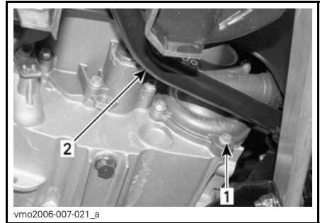
1. Kühlmittelablassschraube 2. Bremspedal
