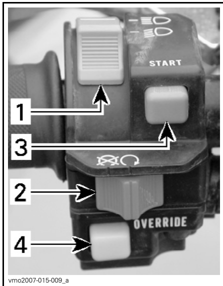
TYPISCH — MULTIFUNKTIONSSCHALTER
