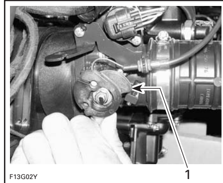
1. Ouverture maximale
