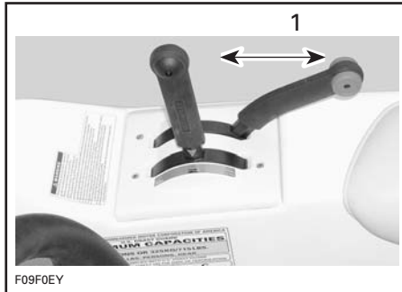
TYPIQUE — LEVIER D'ACCÉLÉRATEUR 1. Doit se déplacer sans entrave
