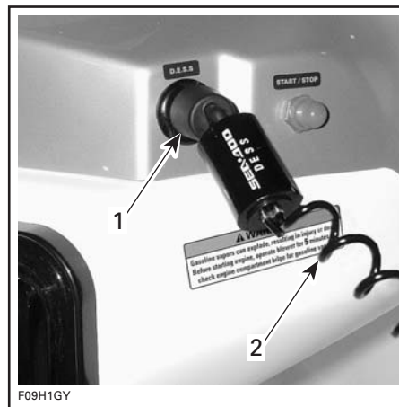
TYPIQUE — INTERRUPTEUR D'ARRÊT ET CORDON DE SÉCURITÉ
