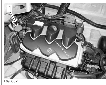
1. Bouchon de remplissage d'huile
