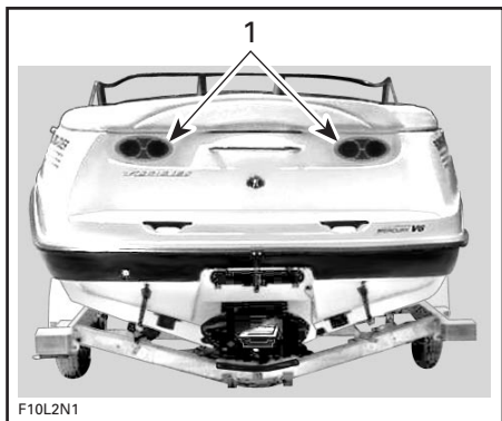
1. Conduits de ventilation de la cale
