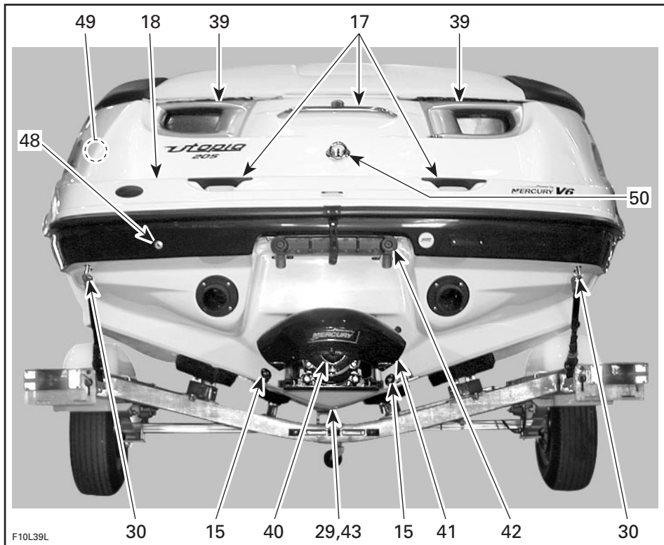
F10L39L TYPIQUE — VUE ARRIÈRE DU UTOPIA 205
