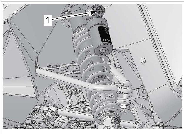
1. 高速圧縮減衰調整装置（六角）
