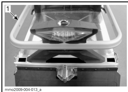
TYPBILD 1. Bakre räckskena
