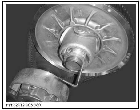
mmo2012-005-980 VARIATORNS UTVIDGARE INSTALLERAD PÅ JUSTERINGSNAVET
