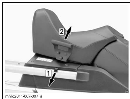
Steg 1: Dra i gummifliken Steg 2: Lyft högra sidan
