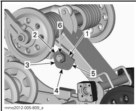
rMOTION OHNE SCHNELLEINSTELLVORRICHTUNG - LINKE SEITE
