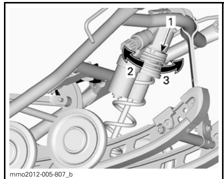
TYPISCH- AUSFÜHRUNG MIT RING 1. Einstellring für Federvorspannung 2. Vorspannung erhöhen 3. Vorspannung verringern
