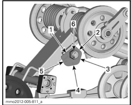
rMOTION OHNE SCHNELLEINSTELLVORRICHTUNG - RECHTE SEITE
