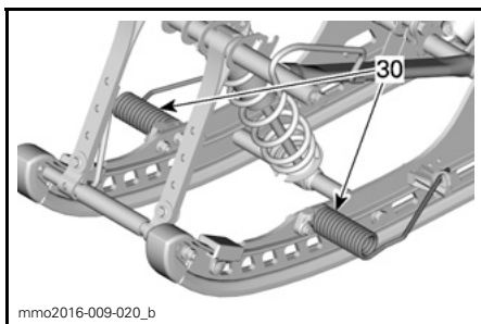
TYPISCH - SUMMIT X MIT T3-PAKET
