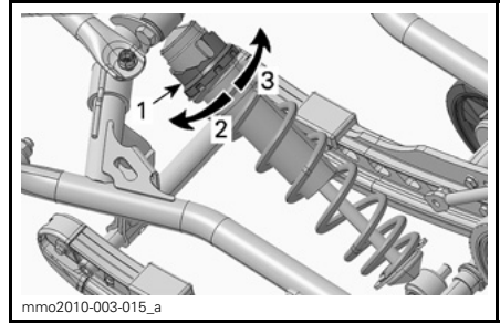
AUSFÜHRUNG MIT NOCKE - HPG™-STOßDÄMPFER 1. Einstellnocke für Federvorspannung 2. Vorspannung verringern 3. Vorspannung erhöhen
