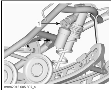
1. Einstellknopf für Kompressionsdämpfung des mittleren Stoßdämpfers
