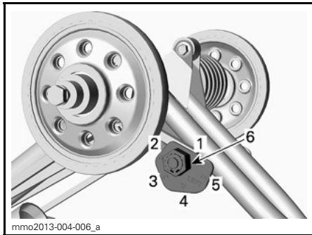
tMOTION - LINKE SEITE
