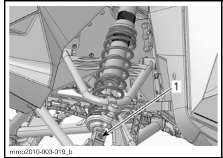
1. Zugstufenverstellung (Knopf)
