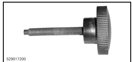
OUTIL D'ÉCARTEMENT DE POULIE MENÉE
