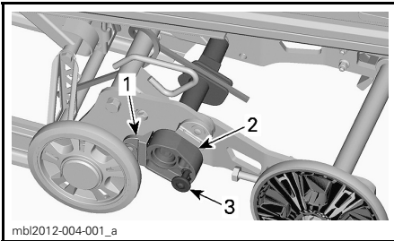
1. Bloc d'arrêt 2. Came stabilisatrice 3. Verrou
