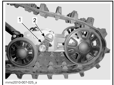
1. Came de réglage 2. Bloc d'arrêt supérieur
