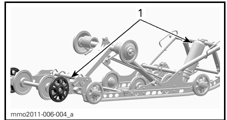
1. Raccords de graissage
