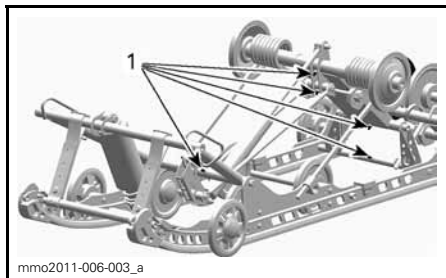
1. Smørenipler
