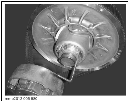
MANDRIN DE POULIE MENÉE SUR UN DISPOSITIF DE RÉGLAGE EN ALUMINIUM
