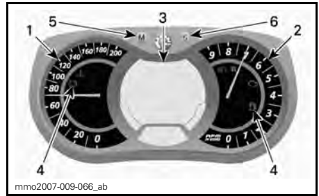
INDICATEUR MULTIFONCTIONNEL ANALOGIQUE/NUMÉRIQUE
