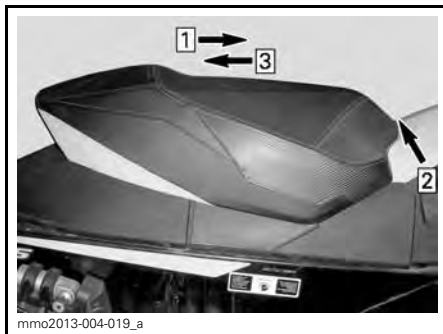
TYPIQUE Étape 1: Pousser le siège vers l'avant Étape 2: Tirer et tenir le verrou Étape 3: Tirer le siège vers l'arrière
