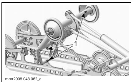
SÉRIES RENEGADE ET GRAND TOURING 1. Raccords de graissage
