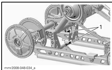
SÉRIES MX Z ET GSX 1. Raccords de graissage
